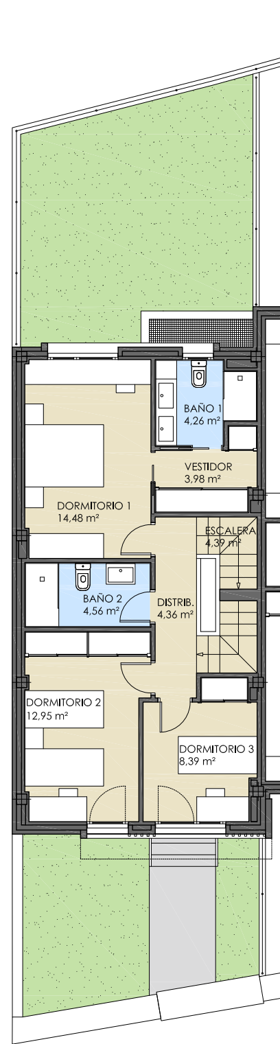
PLANTA PRIMERA
